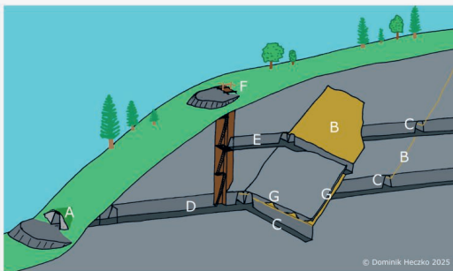
Obrázek 2: Řez idealizovaným dolem na železnou rudu v Nýdku.
